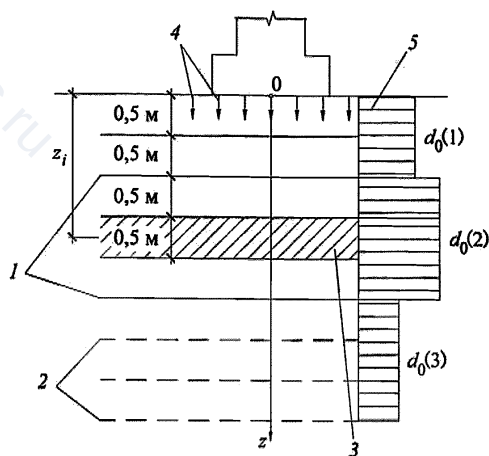
1 – границы слоев с различным содержанием гипса; 2 – границы расчетных слоев; 3 – расчетный слой; 4 – направление фильтрации; 5 – начальная эшпора относительного содержания гипса d_0(z)
