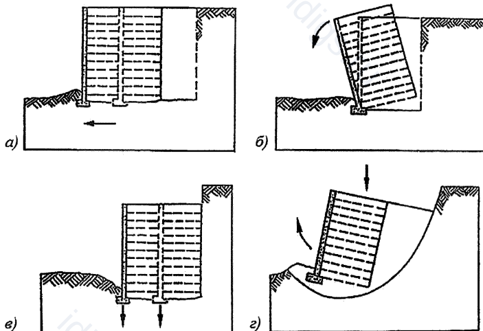
а – сдвиг по подошве; б – опрокидывание; в – потеря несущей способности подстилающего массива грунта; г – глубокий сдвиг
