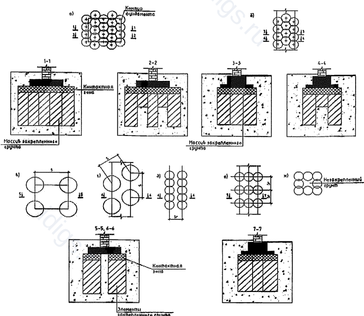
а, б – сплошное из рядов расположенных элементов; в, г – отдельно стоящих элементов; д, е, ж, з – отдельно расположенных рядов сплошных элементов
